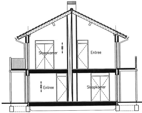
type 6F/6G, doorsnede A-A
